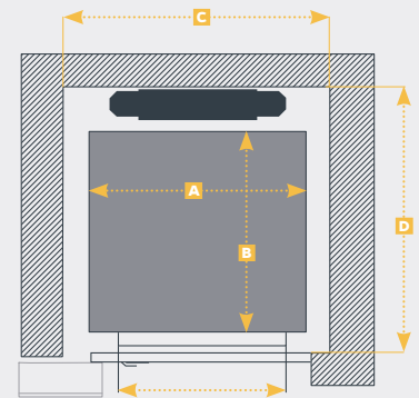
Mécanique Fond de Gaine
